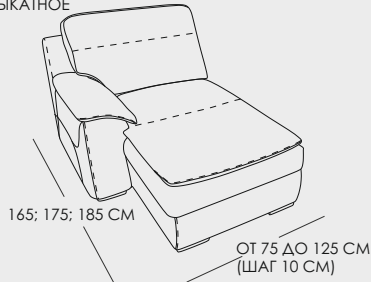
КАНАПЕ: -ЛЕВЫЙ; ПРАВЫЙ - МЕСТО ХРАНЕНИЯ (ПОДЪЕМНЫЙ МЕХАНИЗМ НА ГАЗЛИФТАХ) - ВЫКАТНОЕ
